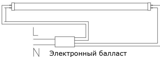
(1) Схема для люминесцентной лампы
